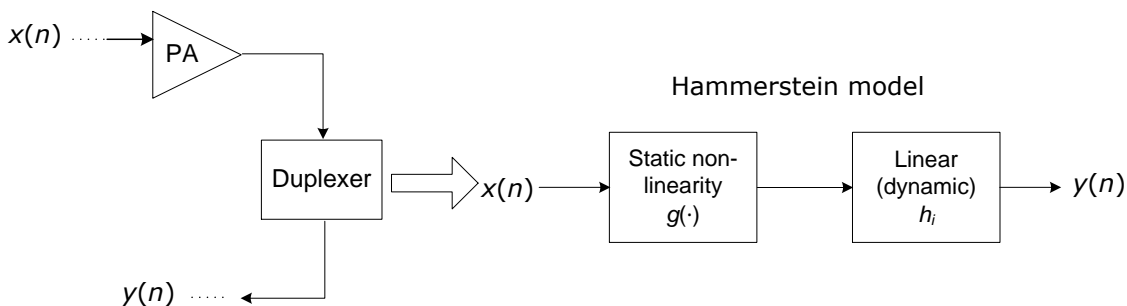
Fig: 2.6. Hammerstein model.
