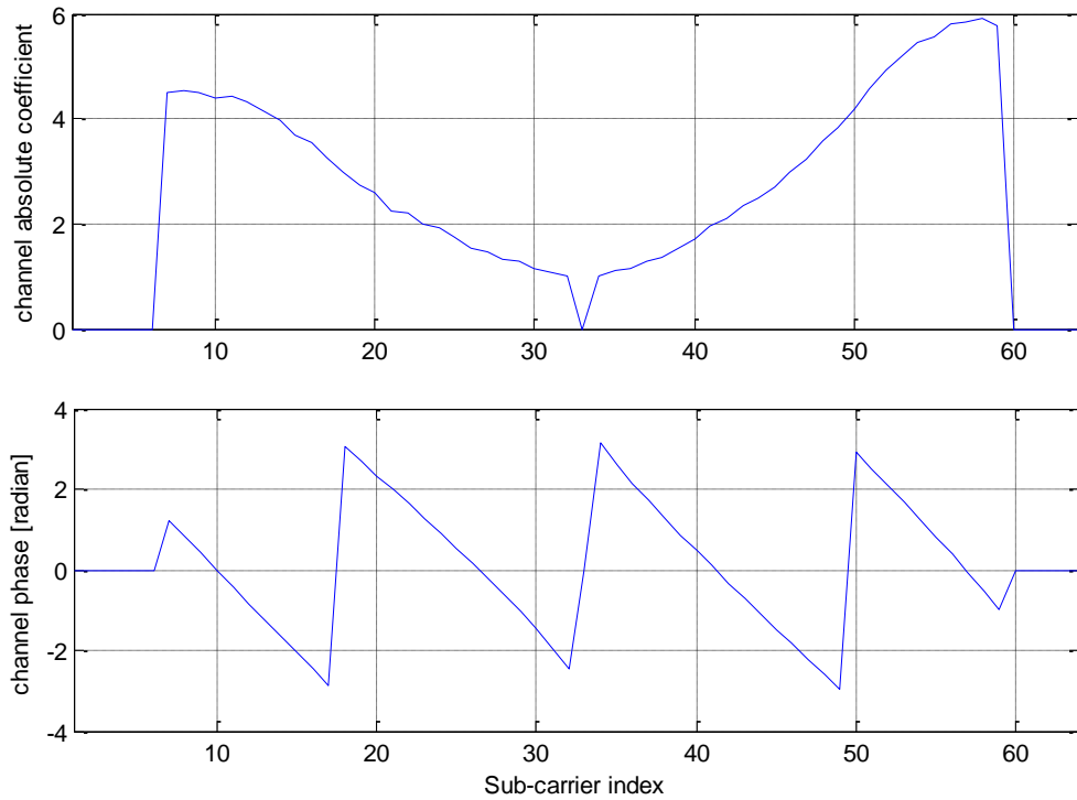
Fig. 5.5. SI channel estimate.
